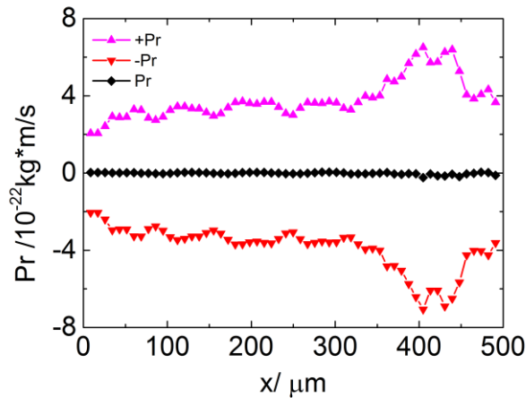
图 4-3 电子的平均方位角动量的演化：粉色的上三角(+Pr)代表正的平均方位角动量（顺时针旋转），红色的下三角(-Pr)代表负的平均方位角动量（逆时针旋转），中间黑色点(Pr)代表总平均方位角动量。
